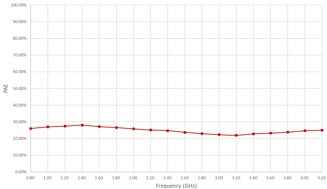
Figure 4: PPA-0080-0420-49 P.A.E
